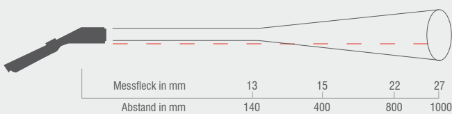
Verhältnis von Entfernung zu Messfleckgröße 20:1
