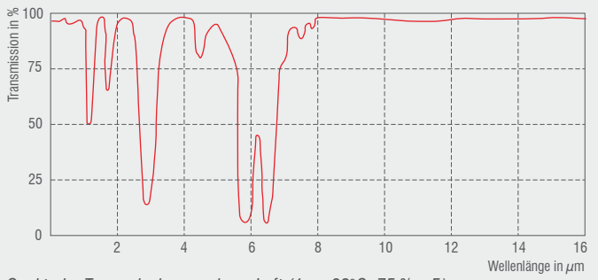
Spektraler Transmissionsgrad von Luft (1 m, 32°C, 75 % r. F.)
