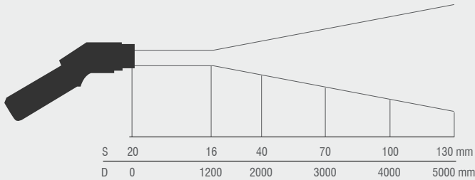
Optisches Diagramm einer Scharfpunktoptik
