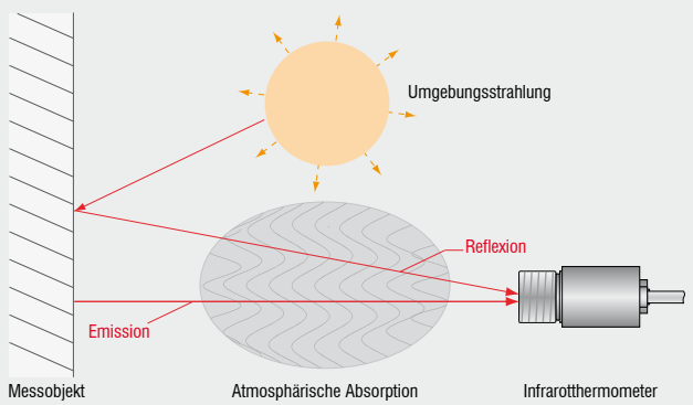
Umgebungsstrahlungskompensation
