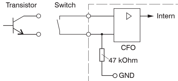
Abb. 16 Beschaltung des Schalteingangs (schematisch)
