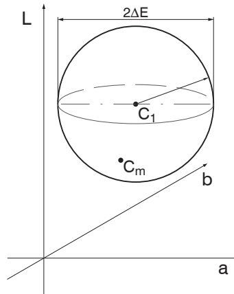
Abb. 2 Toleranzraum Kugel
