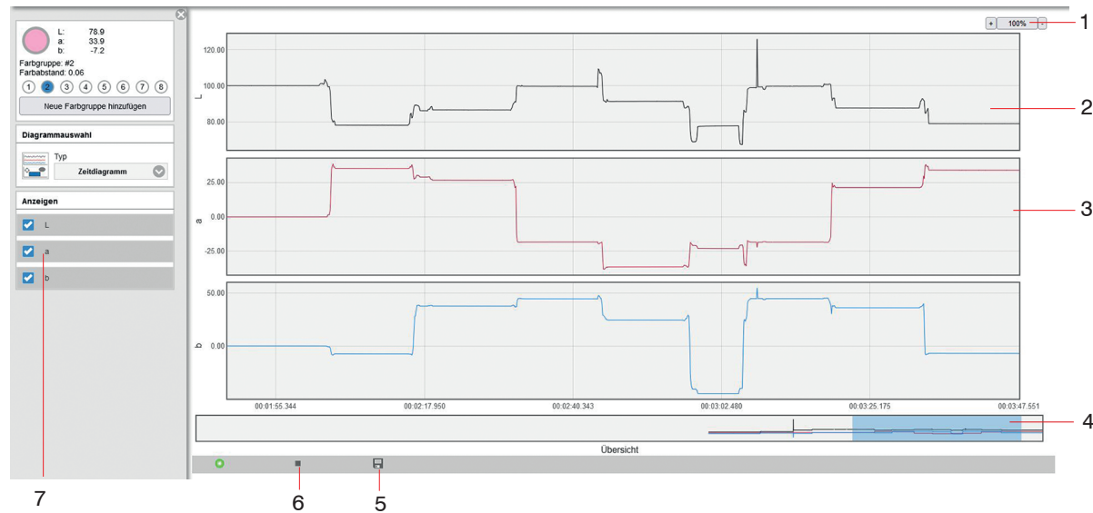
Abb. 32 Ausschnitt Menü Messwertanzeige, Zeitdiagramm
