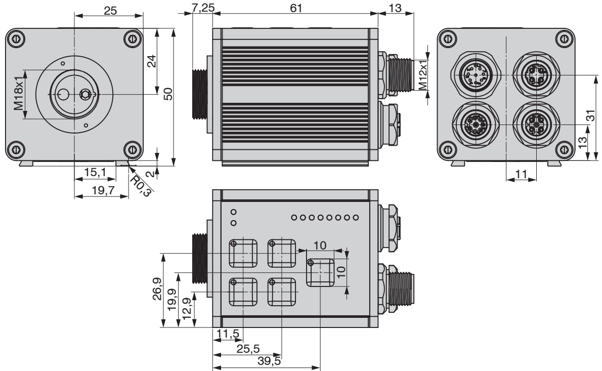
Abb. 6 Maßzeichnung colorSENSOR CFO100/CFO200, Abmessungen in mm
