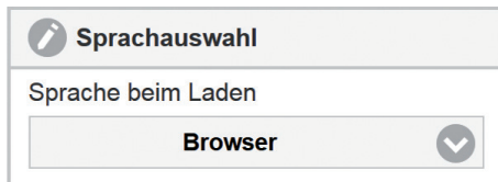
Abb. 57 Ansicht Sprachauswahl
