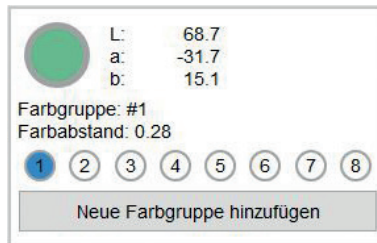
Abb. 28 Fenster Farbanzeige
