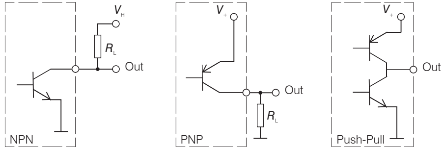
Abb. 17 Beschaltung der Schaltausgänge (schematisch)
