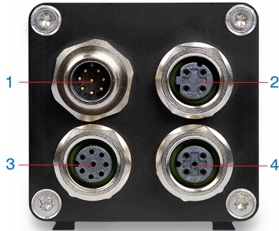
Abb. 10 Buchsenanordnung am colorSENSOR CFO200
