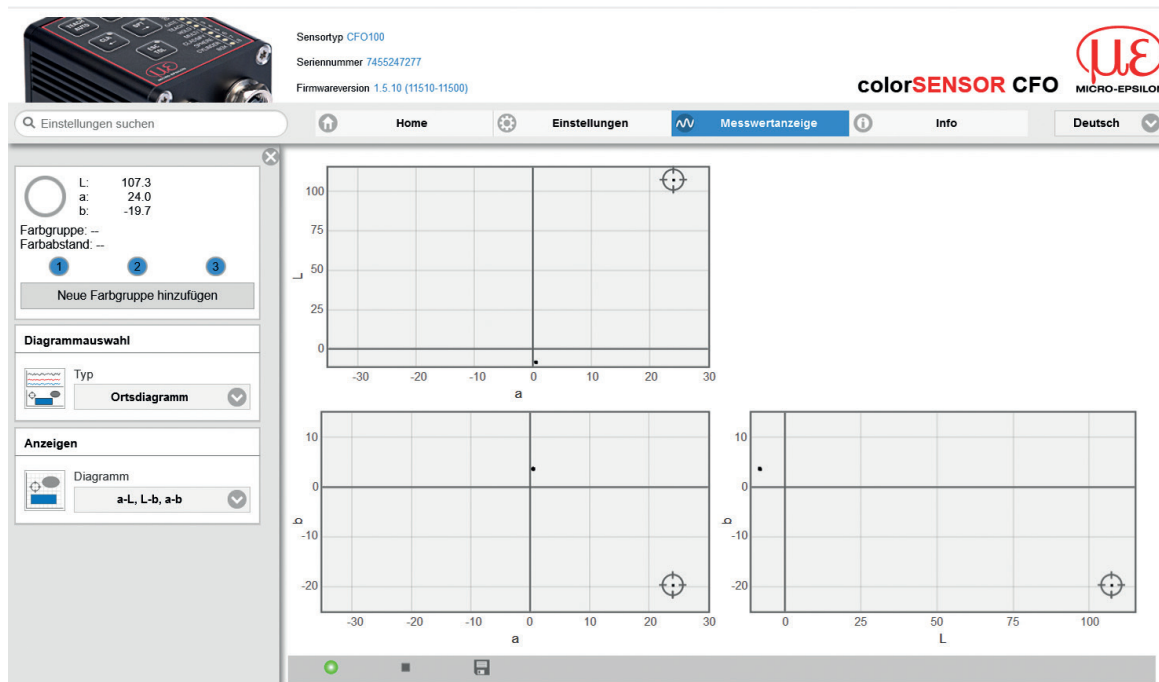
Abb. 66 Ausschnitt Menü Messwertanzeige, Ortsdiagramm
