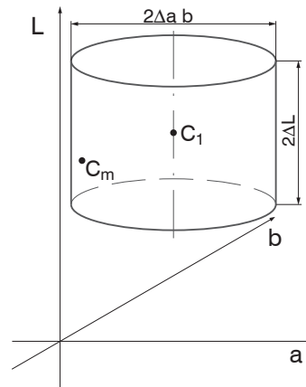
Abb. 3 Toleranzraum Zylinder
