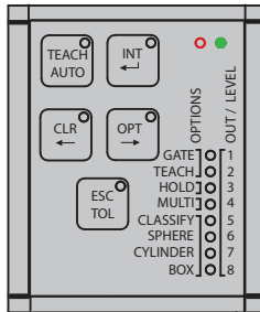
Abb. 23 Ansicht Betriebsmodus
