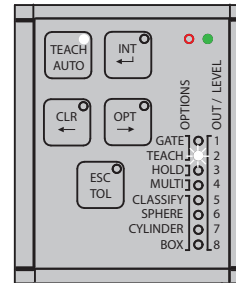
Abb. 24 Ansicht Menümodus
