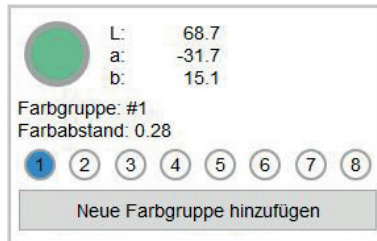
Abb. 46 Fenster Farbanzeige
