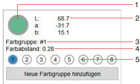
Abb. 33 Ansicht Farbprüfungsanzeige
