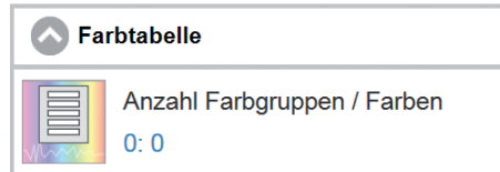
Abb. 44 Fenster Farbtabelle
