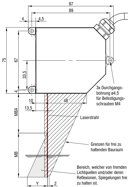
optoNCDT 2300-2 ... 2300-100 Diffuse Reflexion
